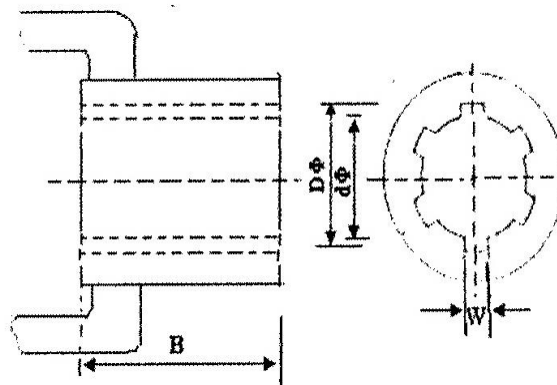
Fig. 2 : Propeller Shaft Insert Dimensions
